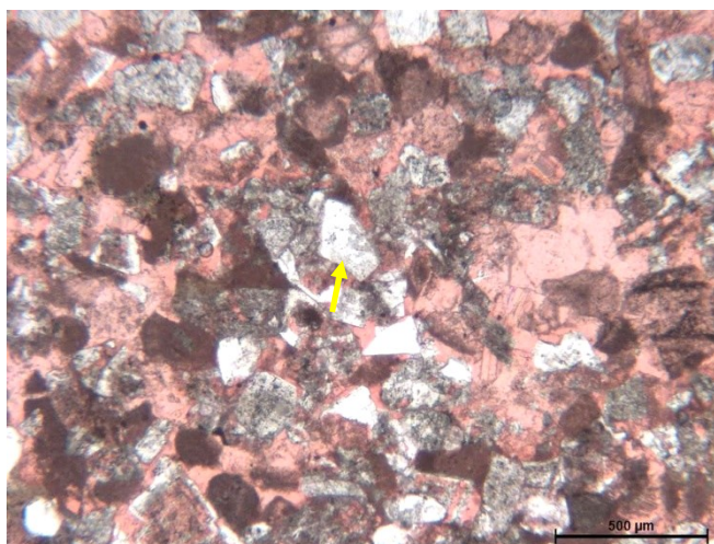
Fig.3. Microfotografía con polarizadores paralelos y tinción de rojo de alizarina, mostrando granos de cuarzo (flecha amarilla). Microphotograph with parallel polarized light, stained with alizarin red, showing quartz grains (yellow arrow).
